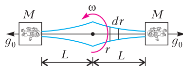
Рис. 3. К определению оптимальной формы троса в системе, вращающейся в невесомости с постоянной угловой скоростью
