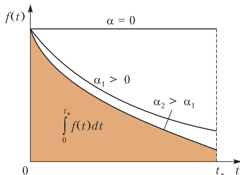
Рис. 3. Зависимость от времени скорости экстракции, учитывающая и ее падение с уменьшающейся температурой (см. рис. 1), и падение самой температуры со временем (см. рис. 2); \alpha — коэффициент теплообмена с окружающей средой. Интеграл по времени от t = 0 до заданного t = t_* — количество экстрагированного вещества
