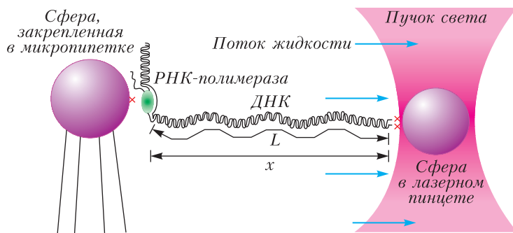
Использование оптического пинцета для изучения структуры РНК-полимеразы
