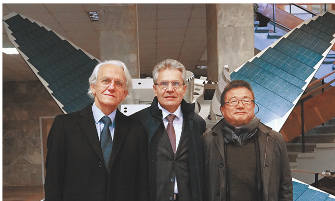
Жерар Муру, Александр Сергеев и Тоси Эбисудзаки на фоне спутника с мощным лазером для уборки космического мусора
