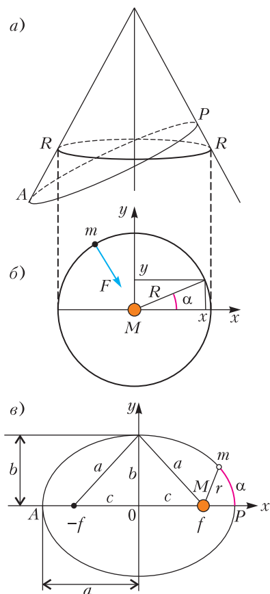
Рис. 3. О конических сечениях. а) Конус, рассеянный плоскостью RR , перпендикулярной его оси, дает окружность радиусом R . Сечение конуса наклонной к его оси плоскостью AP дает эллипс. б) Уравнение окружности – фактически теорема Пифагора для треугольника со сторонами x , y , R ; F – сила тяготения (она же центростремительная), действующая на спутник массой m со стороны гравитирующей массы M . в) Эллипс, в фокусе f которого находится центр гравитации массой M
