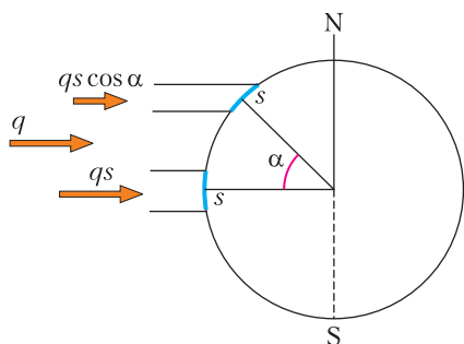
Рис. 4. На одинаковые площадки на поверхности сферы приходятся неодинаковые, в зависимости от \cos \alpha , потоки энергии
