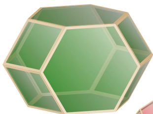
Удлиннный ромбододекаэдр (угол ромба \arccos 1/4 )
