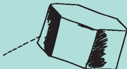
Правильная шестиугольная призма с равными ребрами
