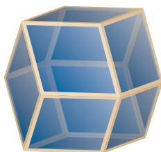
Удлиннный ромбододекаэдр (угол ромба \arccos 1/4 )
