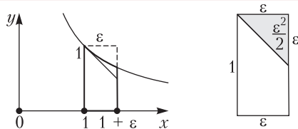
Рис. 11. Приближение для \ln(1 + \epsilon)
