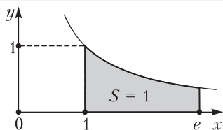
Рис. 10. Определение \epsilon : единичная площадь
