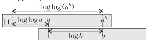
Рис. 7. Возведение в степень
