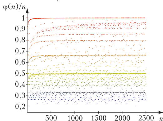
Рис. 1. Значения \varphi(n)/n для n от 1 до 2500
