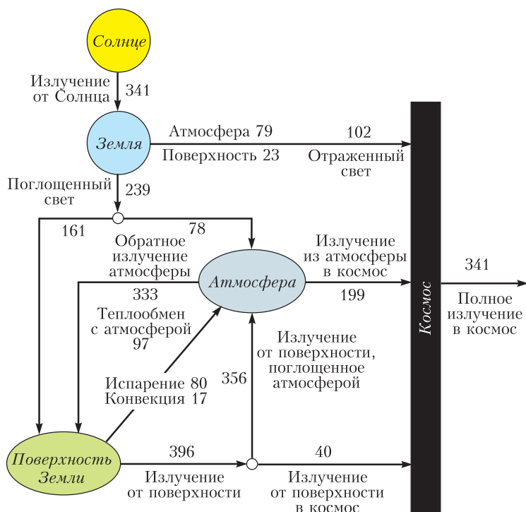
Рис. 1. Тепловой баланс Земли (март 2000 – май 2004). Все тепловые потоки (в \text{Вт}/\text{м}^2 ) усреднены по времени и по поверхности Земли. (Источник: K.T.Trenberth, J.Fasullo, J.T.Kiehl. Earth's global energy budget . – Bull. Amer. Meteor. Soc. , 90 (2009), 311–323.)
