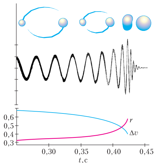
Рис. 2. Слияние пары черных дыр. Верхний ряд – последовательные фазы процесса. Средний – соответствующие колебания напряженности гравитационной волны (условные единицы), полученные в результате численных исследований на основе ОТО. Внизу – изменение со временем расстояния r между звездами и их относительной скорости \Delta v (отнесенной к скорости света)
