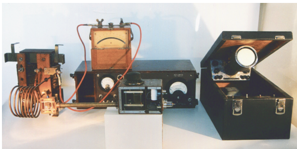
Рис. 6. Экспериментальная установка Е.К.Завойского, 1943–1944 годы
