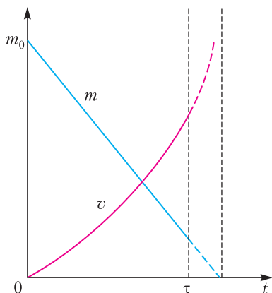
Рис. 1. Ракета ускоряется за счет отбрасывания назад только собственной массы, ее скорость и ускорение могут достичь произвольно заданной величины
