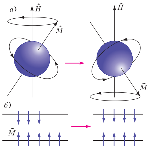
Рис. 4. Иллюстрация переходов между состояниями с разными ориентациями дипольного момента частицы \vec{M} относительно внешнего магнитного поля напряженности \vec{H} в терминах классической (а) и квантовой (б) физики. В обоих случаях переход обозначен красной стрелкой
