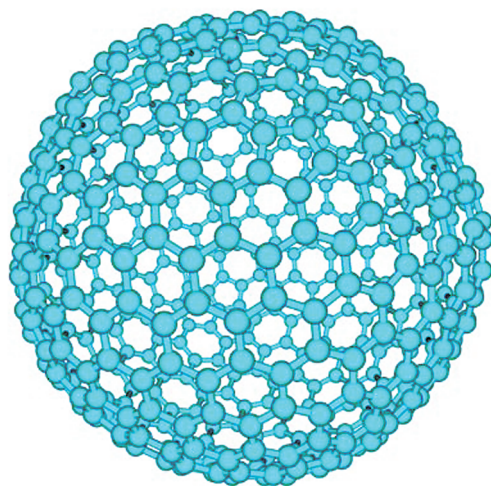
Рис. 6. Молекула C_{540}
