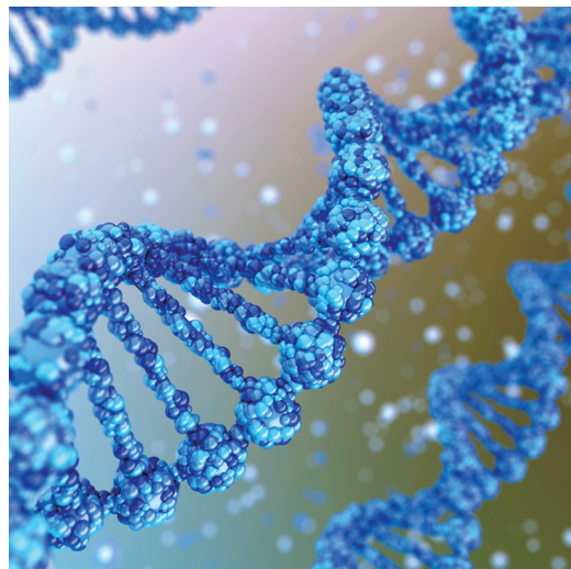
Рис. 1. Двойная спираль молекулы ДНК (дезоксирибонуклеиновой кислоты), которая кодирует генетическую информацию. Структура ДНК была выявлена с помощью рентгеновской дифракции. Молекула состоит из четырех типов нуклеотидов, которые комплементарно собраны на каждой нити, что дает ей возможность реплицироваться (возобновляться)
