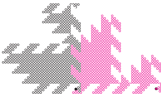
Рис. 15. Здесь одна из двух половин кривой (она называется «Паровоз») нарисована цветной, чтобы показать, как эти две кривые «сцепляются» между собой. Одна половина после поворота ее вокруг средней точки на 90^\circ совпадет с другой
