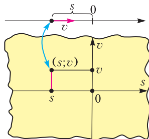
Рис. 1. Движение по прямой
