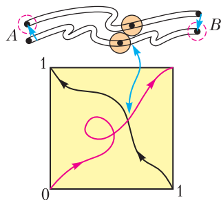
Рис. 3. Задача о двух возах на двух дорогах
