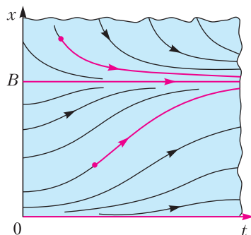
Рис. 9. Решения уравнения отлова с относительной квотой \dot{x} = (1-x)x - px при p < 1 . Любая популяция стремится к устойчивому значению x = B
