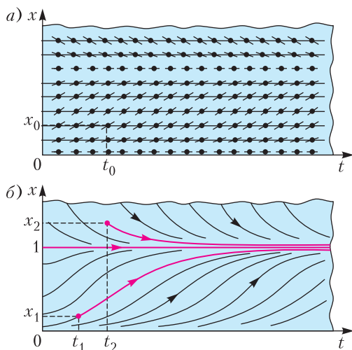
Рис. 7. Поле направлений и графики решений логистического уравнения \dot{x} = (1 - x)x . Решения x = 1 и x = 0 отвечают положениям устойчивого и неустойчивого равновесия
