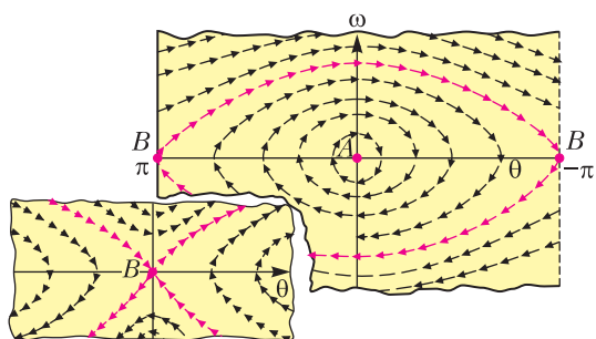
Рис. 5. Поле фазовой скорости математического маятника
