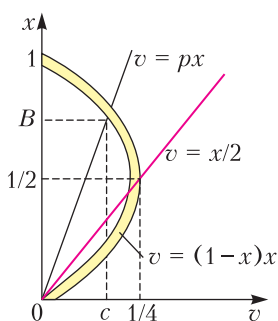
Рис. 10. Нахождение оптимального устойчивого режима отлова c относительно квотой
