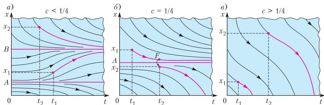
Рис. 8. Решения уравнения отлова \dot{x} = (1-x)x - c при разных значениях квоты отлова c . При c < 1/4 любая популяция стремится к устойчивому равновесию x = B , при c = 1/4 положение равновесия неустойчиво, при c > 1/4 любая популяция вымирает
