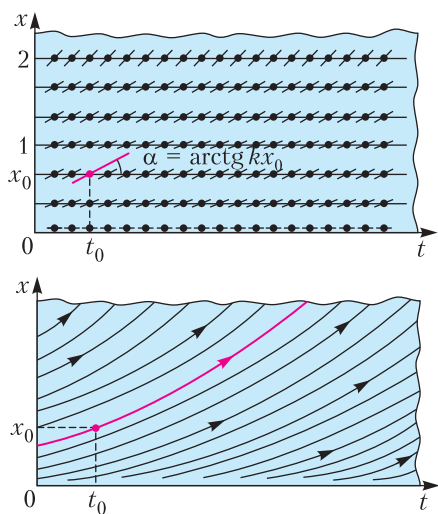
Рис. 6. Поле направлений уравнения нормального размножения \dot{x} = kx и решение, проходящее через начальную точку (t_0; x_0)
