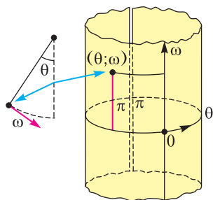
Рис. 2. Колебания маятника
