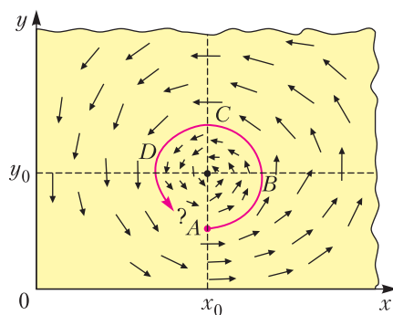
Рис. 11. Поле фазовой скорости в модели «хищник–жертва»
