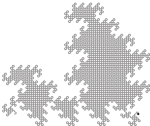
Рис. 14. Эта кривая дракона ранга 12 имеет специальное название «Папа, мама и сын». Найдите ее середину. Можете ли вы себе представить, что кривая разбивается этой точкой на два совершенно одинаковых куска, получающихся друг из друга поворотом на 90^\circ ? Чтобы поверить в это, придется, вероятно, пройтись по кривой цветным карандашом от начала до середины
