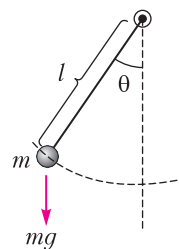
Рис. 4. Математический маятник
